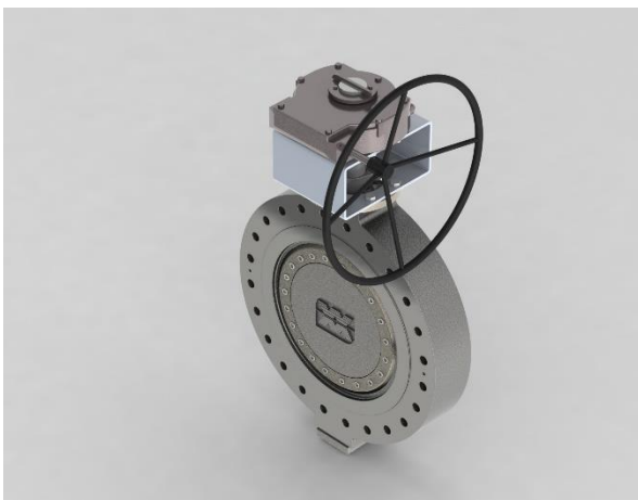
Klappe in Anflanschausführung mit Handgetriebe
